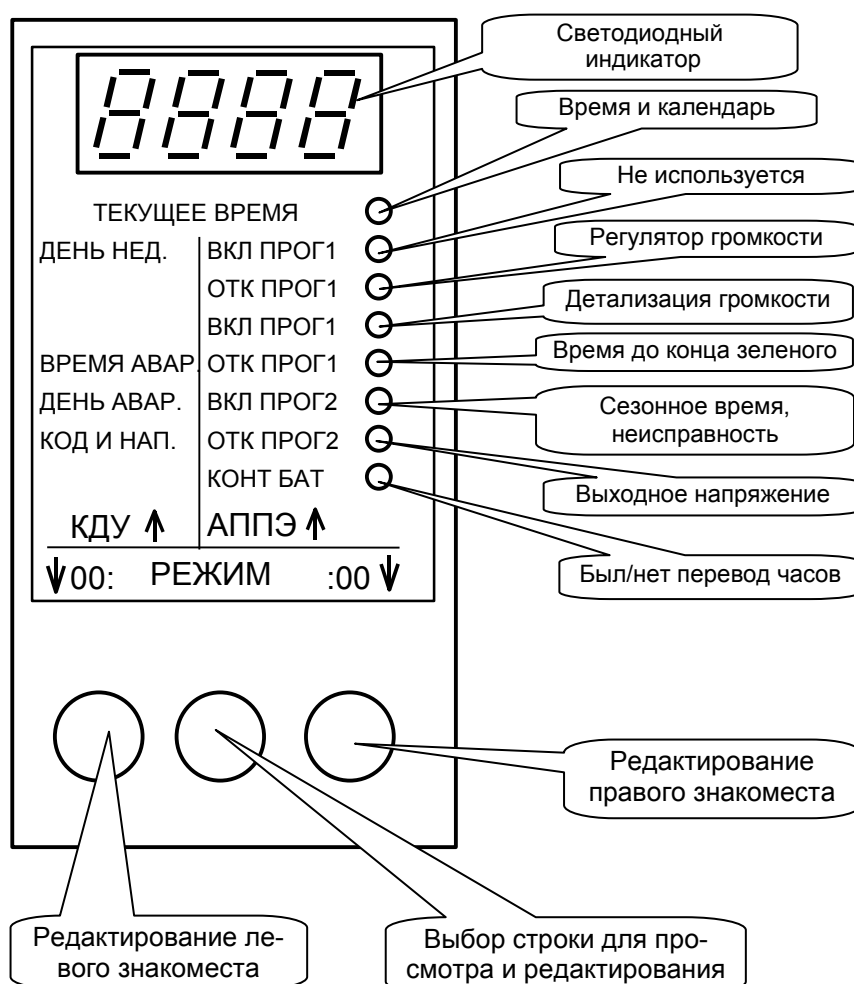
Назначение строк и кнопок пульта ПД-2 при работе с УЗС-1(М)
