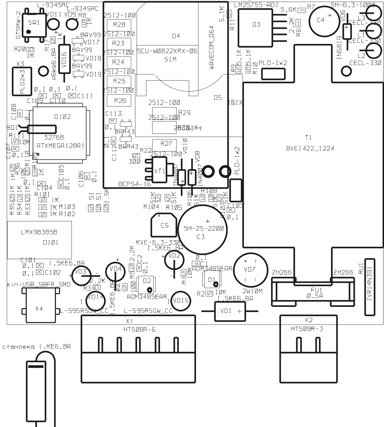
ММС-04 изм. 1. Внешний вид платы со стороны элементов.
